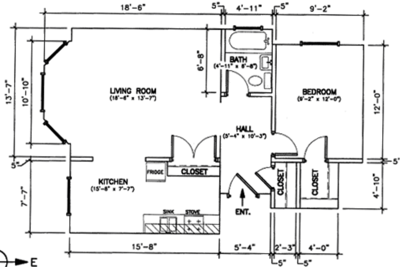
APT. 501 6151 N. WINTHROP SCALE: 3/16"=1'-0"
